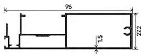
INTERLOCK
