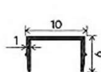
CLIP
