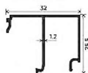
CLIP
