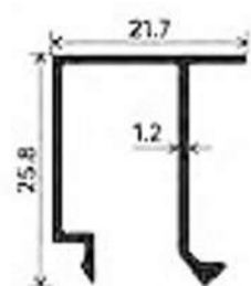
CLIP
