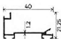
ECO CLIP
