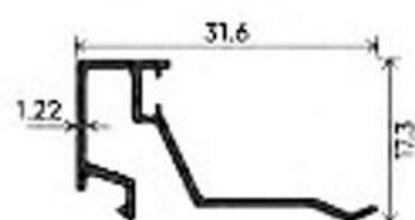
INTERLOCK CLIP
