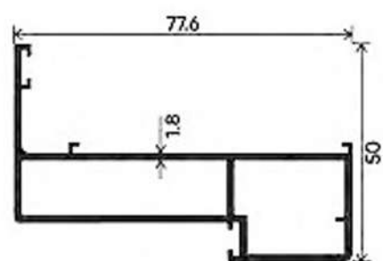
DOOR FRAME
