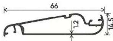
LOUVER SECTION
