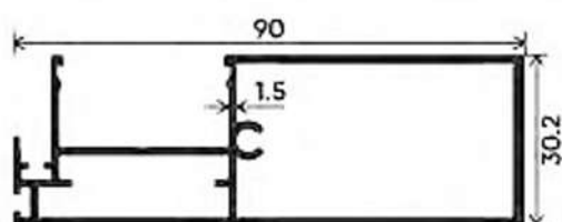
INTERLOCK
