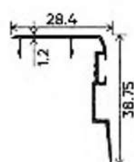
CLIP
