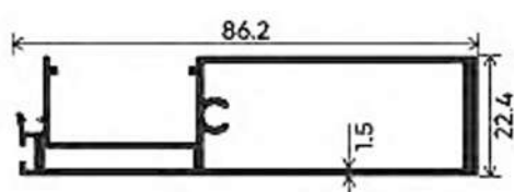
CLIP
