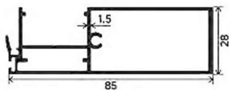
INTERLOCK
