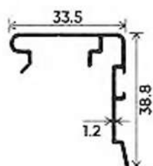
INTERLOCK CLIP
